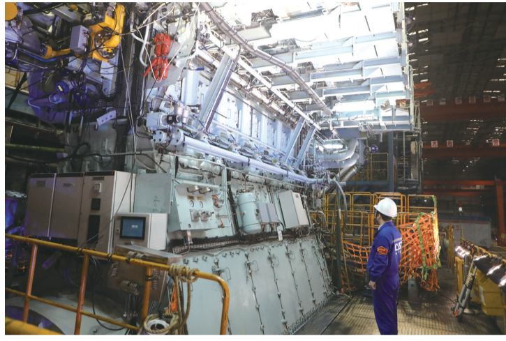
我国首台自主研发全球最小缸径双燃料低速发动机(CX40DF)在江苏镇江中船动力交付。
